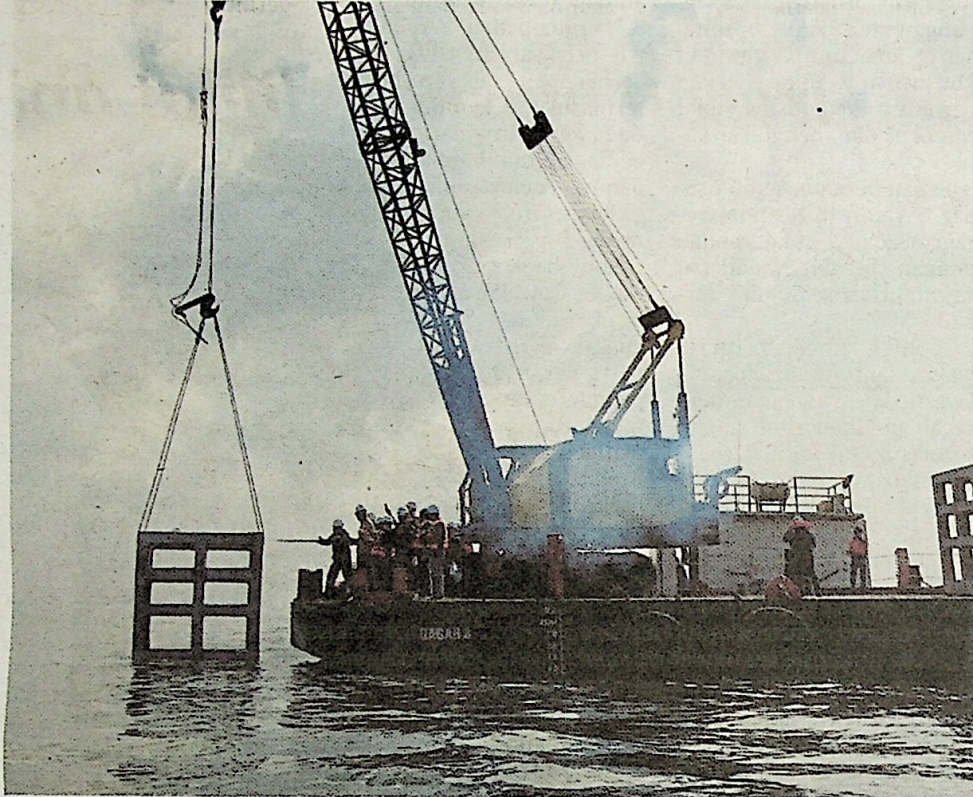
PROSES melabuhkan tukun tiruan konkrit di perairan Pulau Nangka. Gambar - NSTP/NURALIAWATI SABRI.
